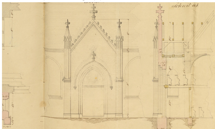
2. Kościół p.w. św. Michała Archanioła w Karlinie. Projekt wejścia bocznego od strony południowej wykonany przez W. Beilke w 1871 r.
